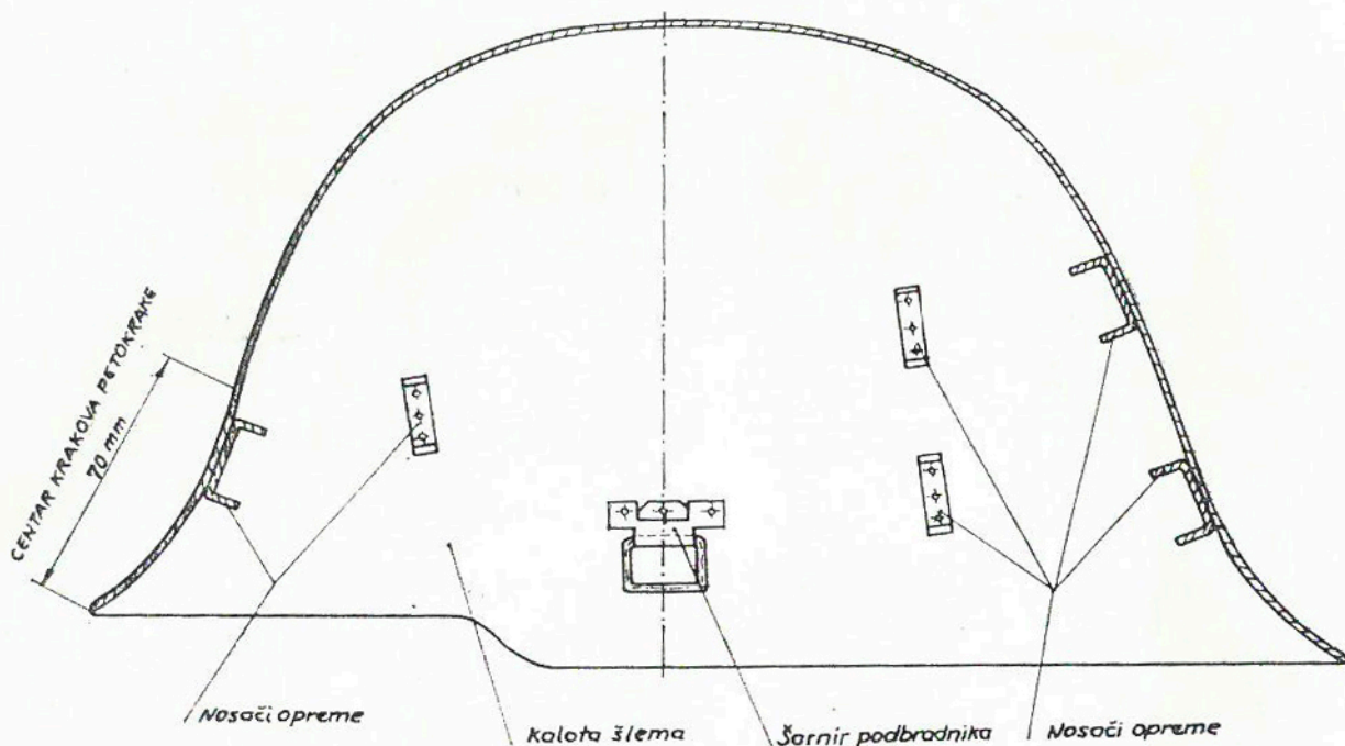
Sl. 2 — Kalota šlema M59 (presek)
