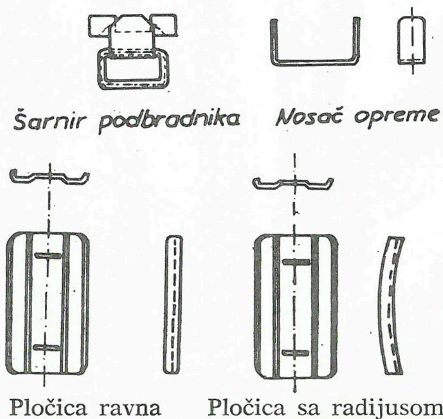
Sl. 3 — Delovi za utvrđivanje opreme šlema M59
