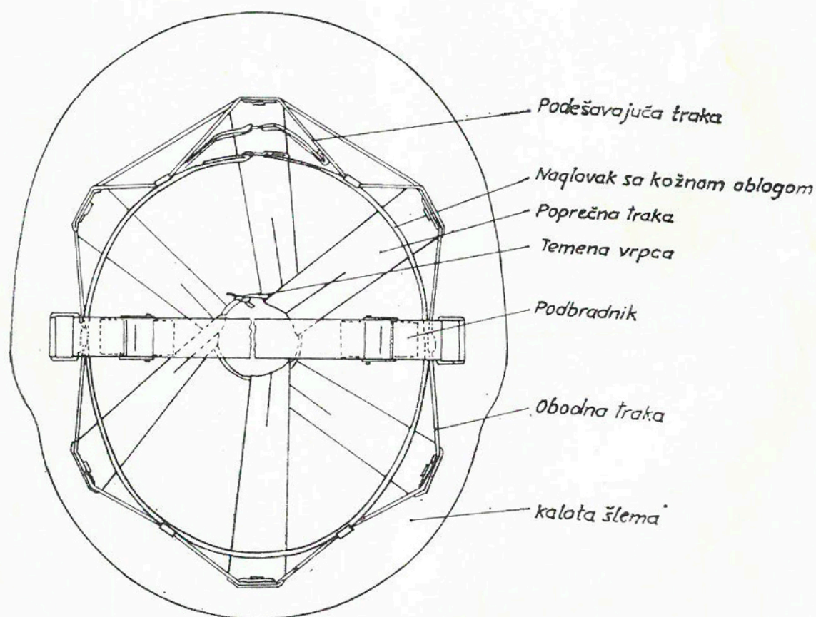
Sl. 5 — Unutrašnja oprema šlema
